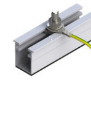
Befestigung des Erdungdrahts mittels Hammerkopfschraube
